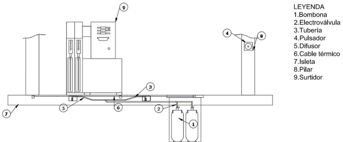
Figura 1: Disposición de los elementos del sistema KIT PETCI, en alzado
