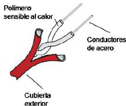
Figura 8.- Descripción de la configuración del cable térmico
