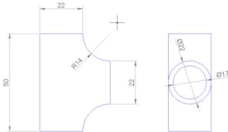
Figura 5.- Planos descriptivos del T. Cotas en mm
