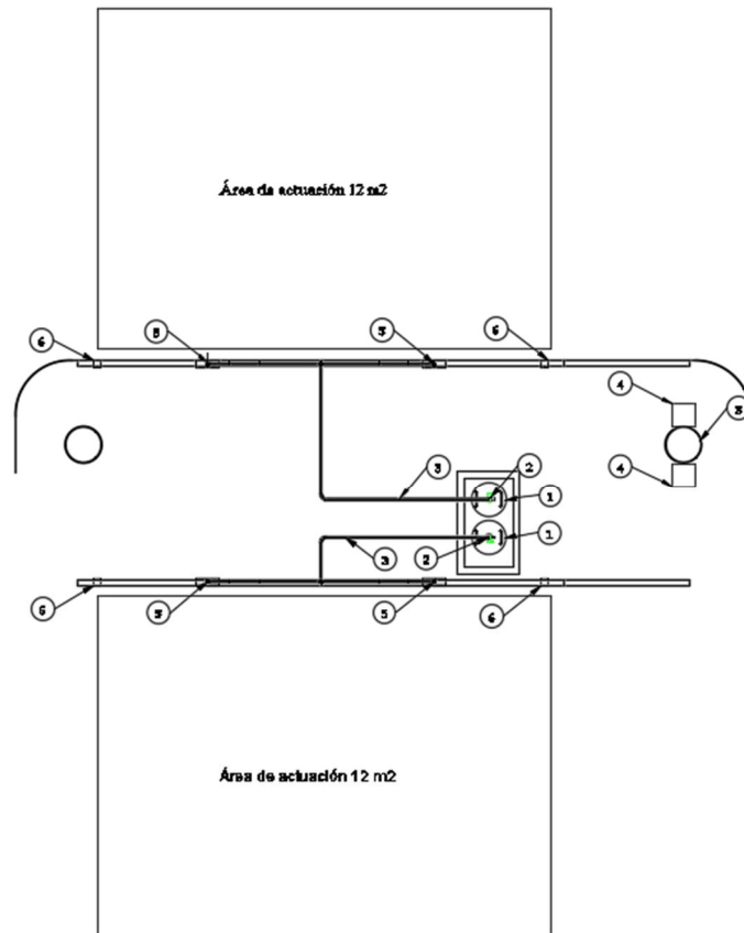
Figura 2: Disposición de los elementos del sistema KIT PETCI, visto en planta
